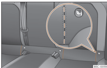
Sl. 27 Stražnje sjedalo: urezani prorezi za pristup ISOFIX/i-Size pričvršnim ušicama.
