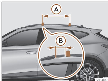
Sl. 123 Pričvršne točke uzdužnih nosača za krovni nosač prtljage.
