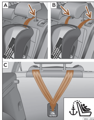
Sl. 29 Stražnja sjedala: namještanje i ugradnja ovisno o Top Tether pojasu.
