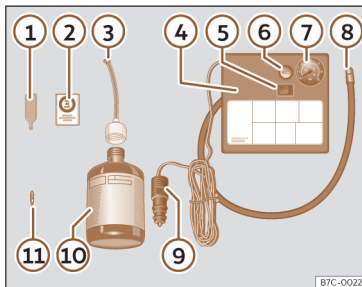
Sl. 34 Prikaz principa: sastavni dijelovi kompleta za popravak guma.
