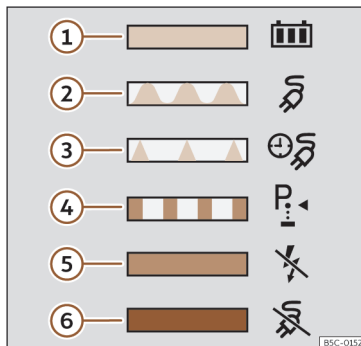
Sl. 196 Na unutrašnjoj strani poklopca priključka za punjenje baterije: naljepnica s informacijama o pokazivaču postupka punjenja.
