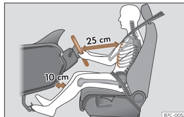
Sl. 2 Pravilan razmak vozača od kola upravljača mora iznositi barem 25 cm (10 inča).
