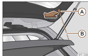
Sl. 111 U prtljažniku: demontiranje i montiranje pokrivke prtljažnika.
