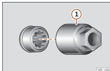
Sl. 36 Vijci kotača sa zaštitom od krađe s poklopcem i adapterom
