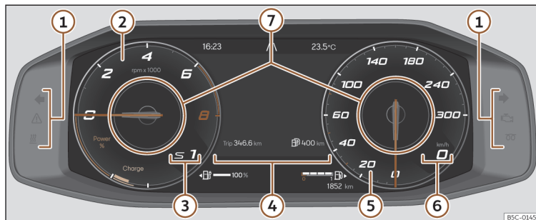
SI. 52 Digital Cockpit u instrumentnoj ploči (klasični prikaz).
