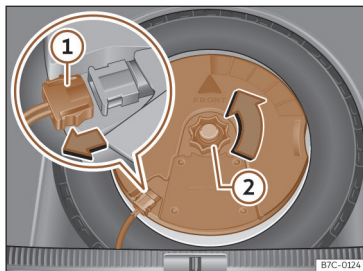
Sl. 224 U prtljažniku: demontiranje subwoofera.
