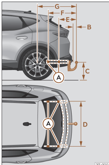
Sl. 189 Dimenzije i pričvrсна mjesta za naknadnu ugradnju mehanizma za vuču
