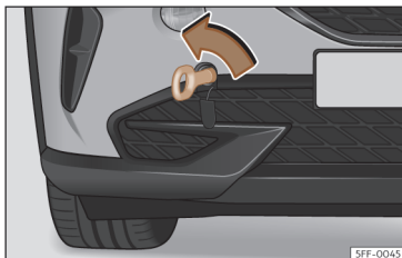
Sl. 44 Branik sprijeda desno: zavrnutu ušicu za vuču.
