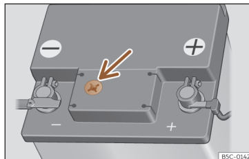
Sl. 218 Prozorčić na gornjoj strani 12-V akumulatora vozila (prikaz principa).
