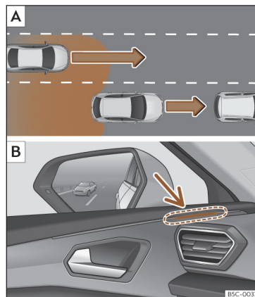
Sl. 170 Shematski prikaz: A Pretjecanje s prometom u stražnjem području. B Prikaz potpore pri promjeni voznog traka na lijevoj kontrolnoj žaruljici.
