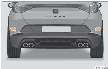
Sl. 151 Prikaz vozila straga: područja radarskih senzora.
